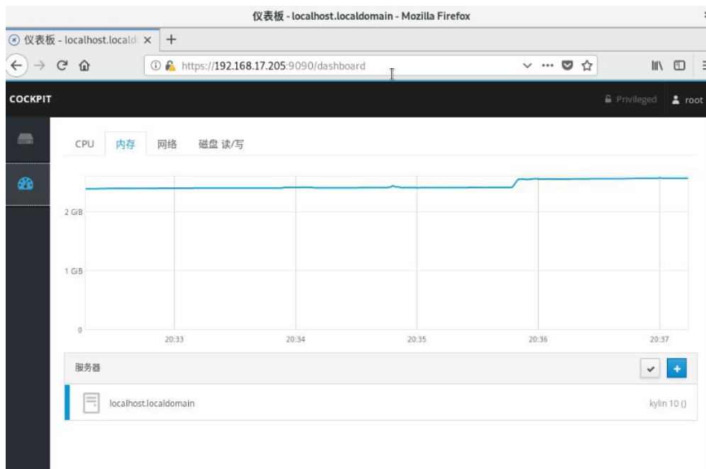
图 3-27 仪表盘界面
