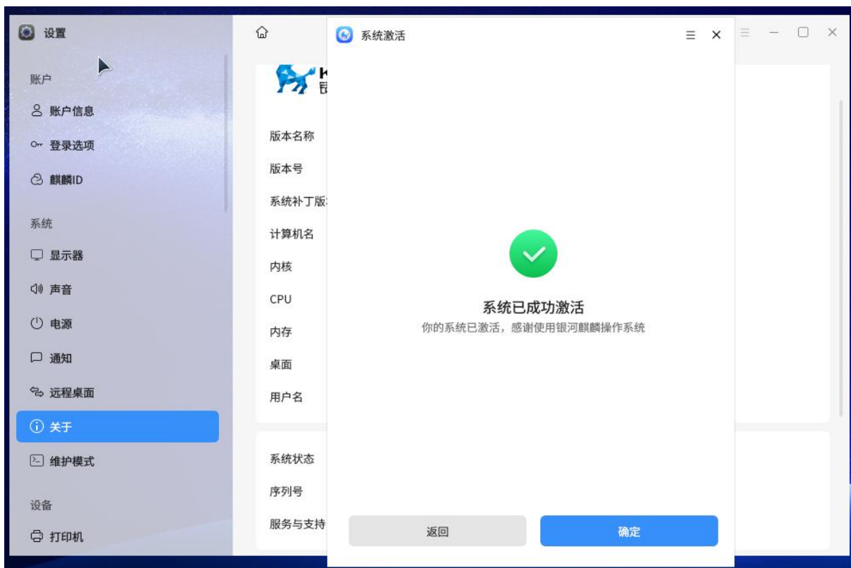
图 5 激活成功
