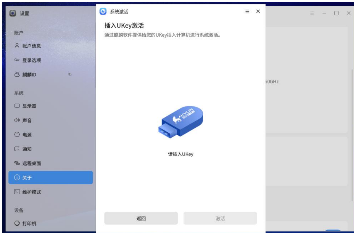
图 21 Ukey 激活
