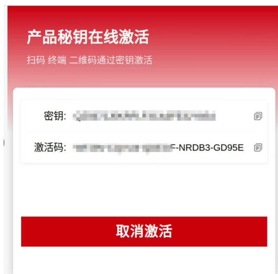
图 9 获取激活码
