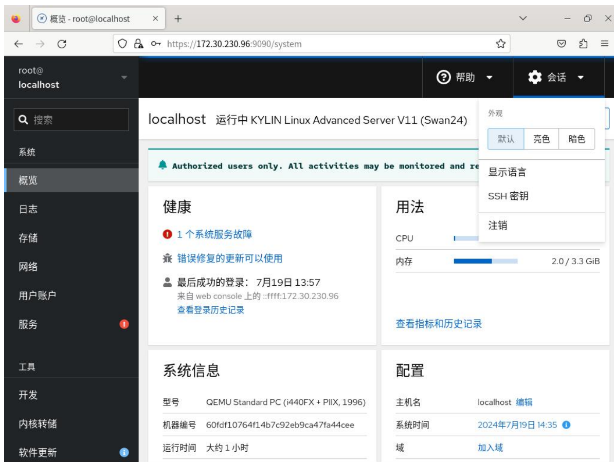
图 4-7 语言切换
