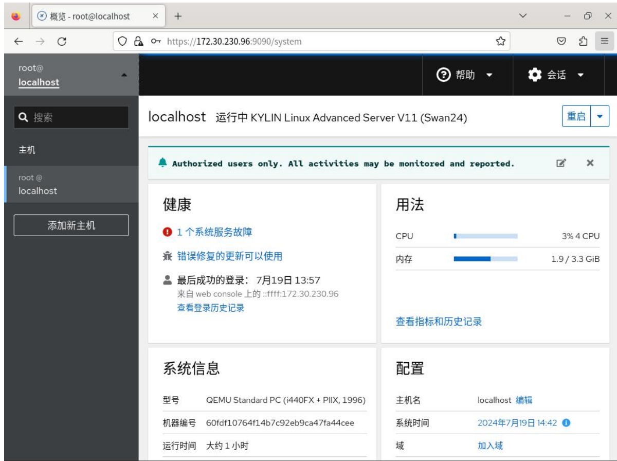
图 4-14 仪表盘界面
