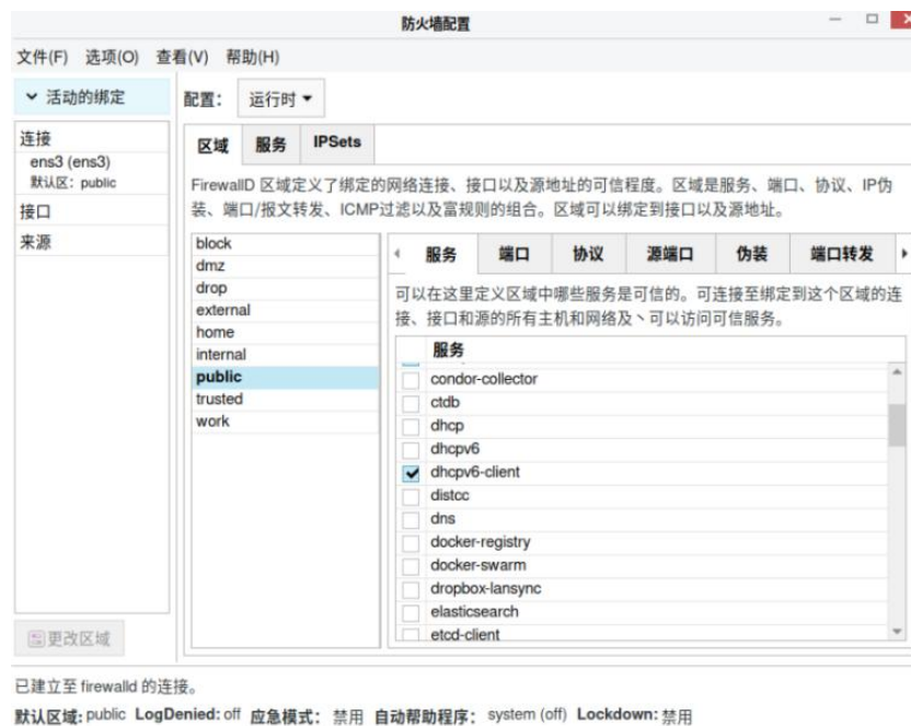
图 9-2 服务选项卡
