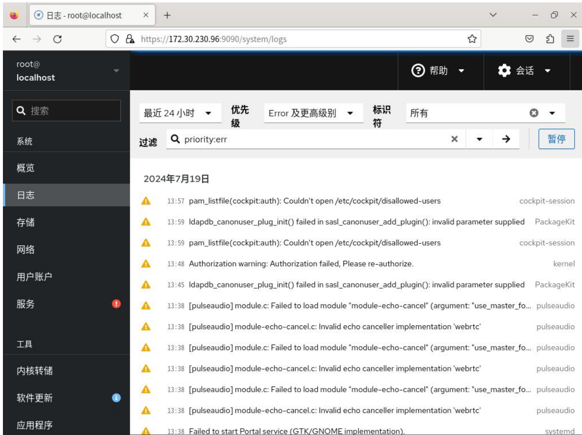
图 4-10 日志界面
