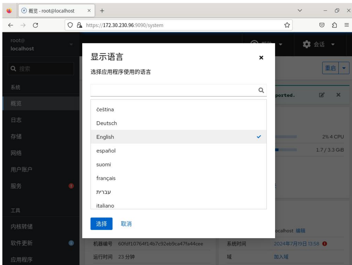
图 4-8 语言选择
