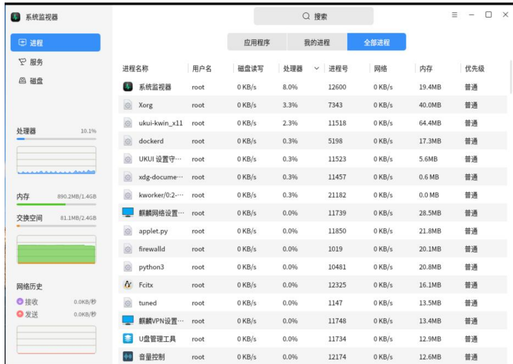
图 8-1 进程
