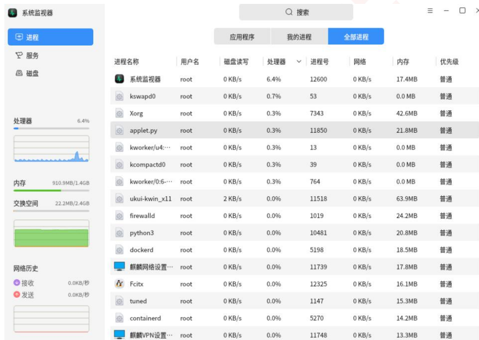
图 8-2 系统监视器
