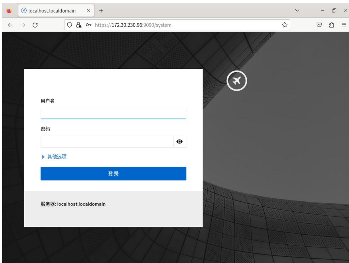
图 4-5 登录界面
