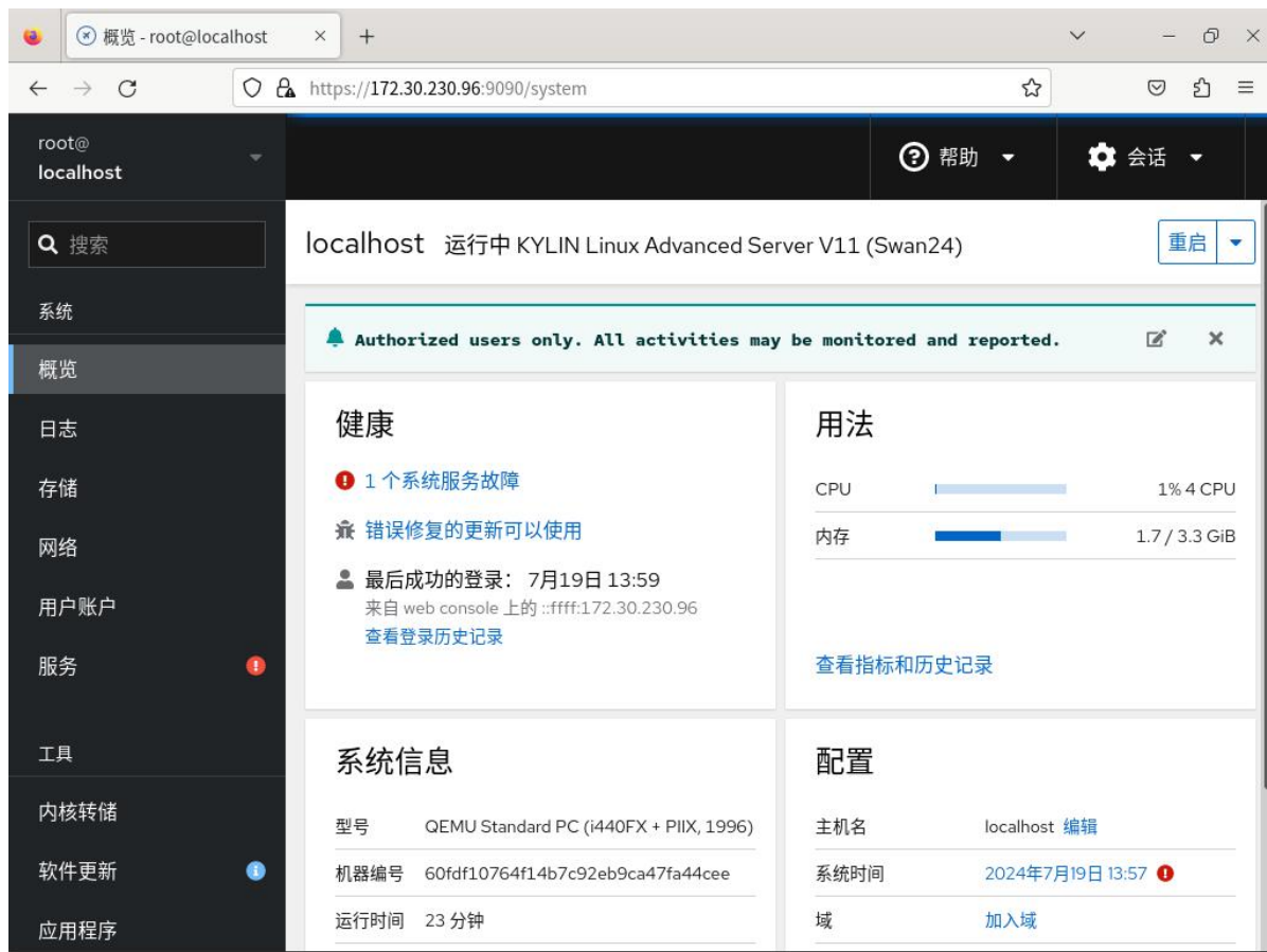
图 4-6 登录后界面
