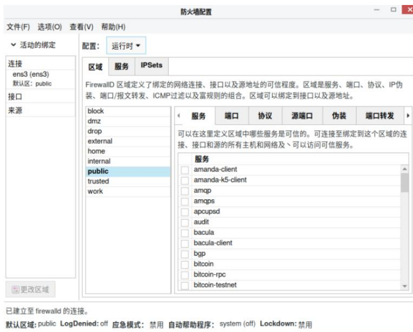
图 9-1 防火墙配置
