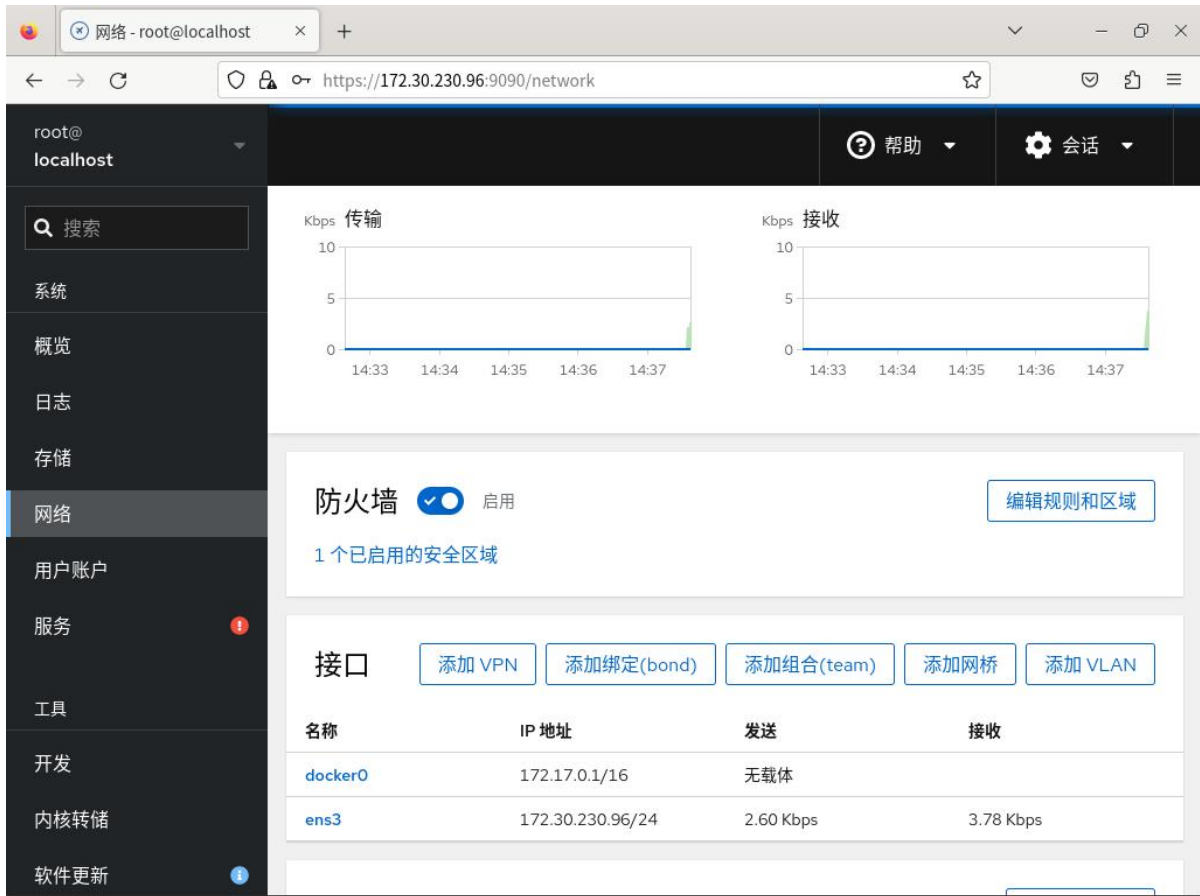
图 4-11 网络界面
