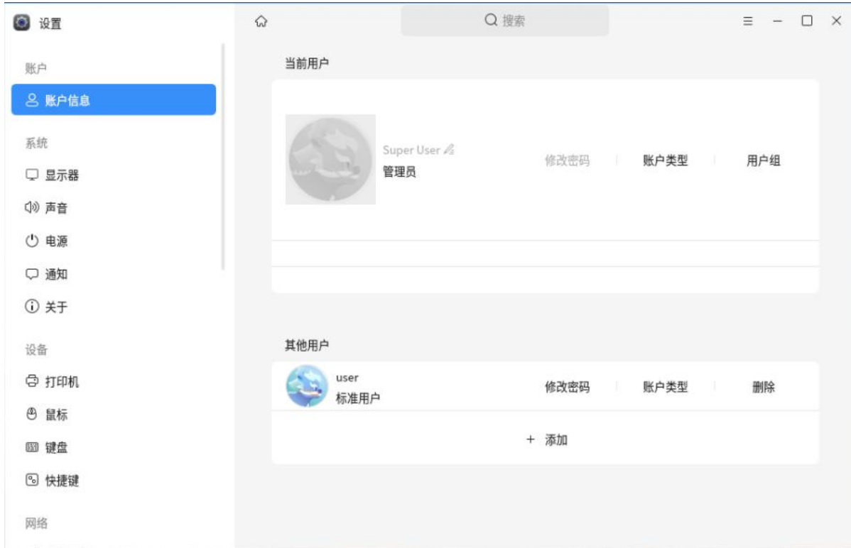
图 2-2 用户账户
