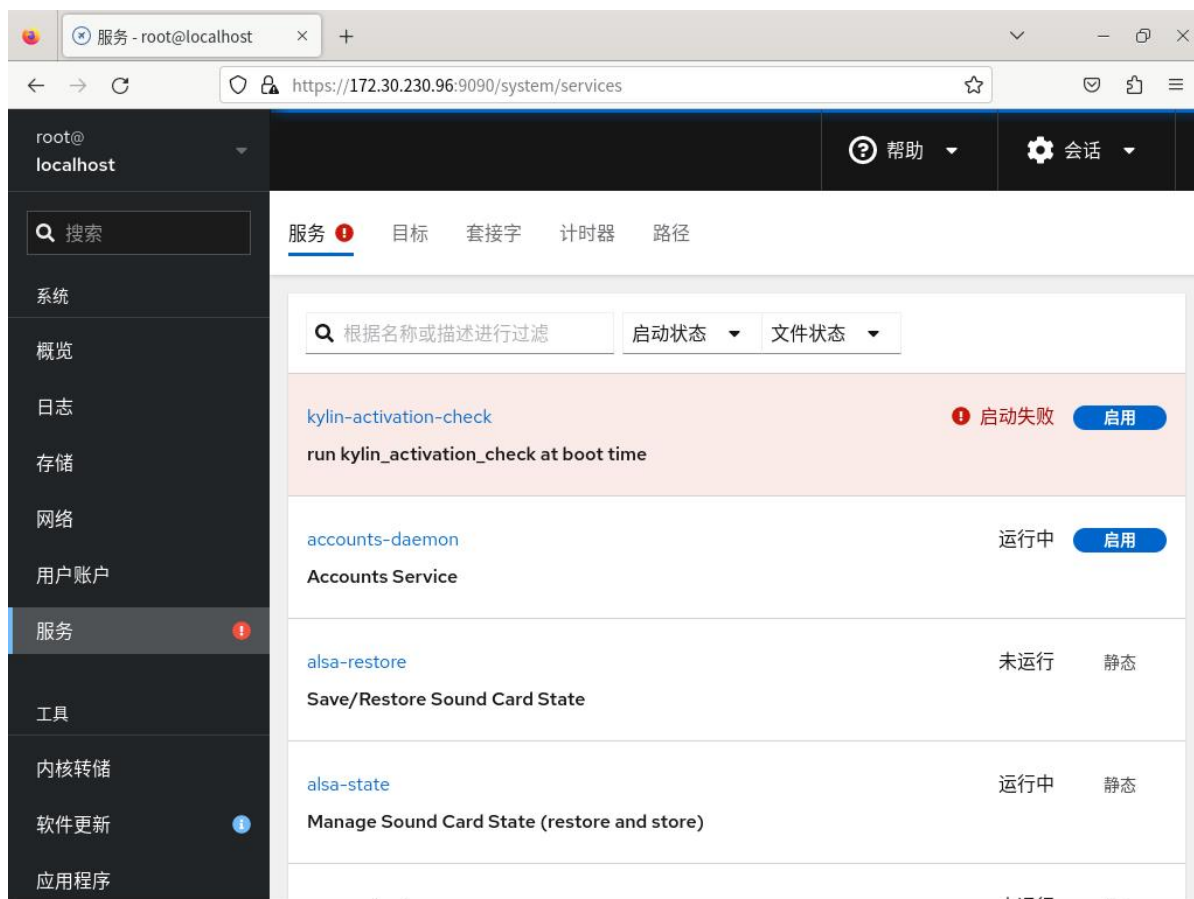
图 4-12 服务界面
