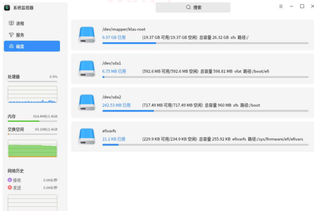
图 8-3 磁盘空间
