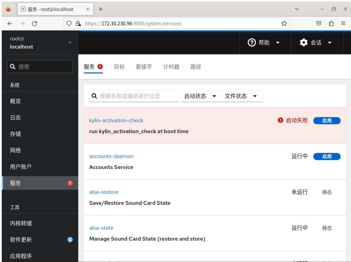
图 4-13 终端界面
