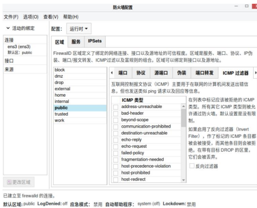
图 8-6ICMP 过滤器子选项卡
