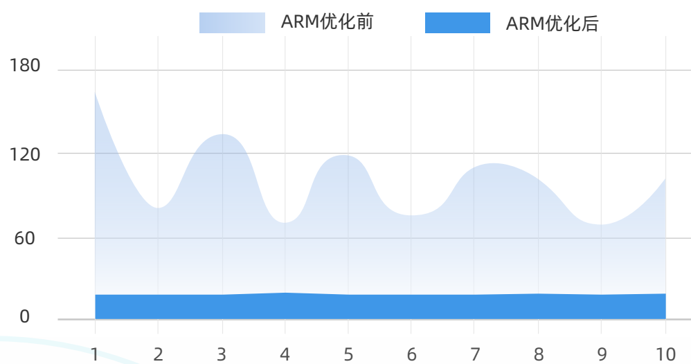
ARM-iSCSI 链路切换时间优化（单位:秒）
