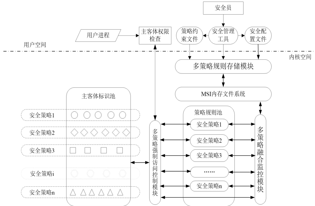
图 2-9 多策略融合控制总体流程
